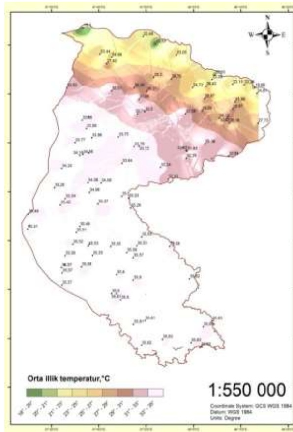
Şəkil 2. İnterpolyasiya metodu ilə orta illik tempratur məlumatlarının ərazi üzrə paylanması xəritəsi (İDW)
