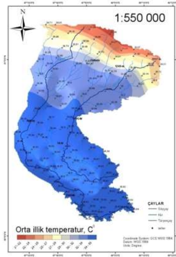
Şəkil 3. İnterpolyasiya metodu ilə orta illik tempratur məlumatlarının ərazi üzrə paylanması xəritəsi (Kriking metodunun tətbiqi )
